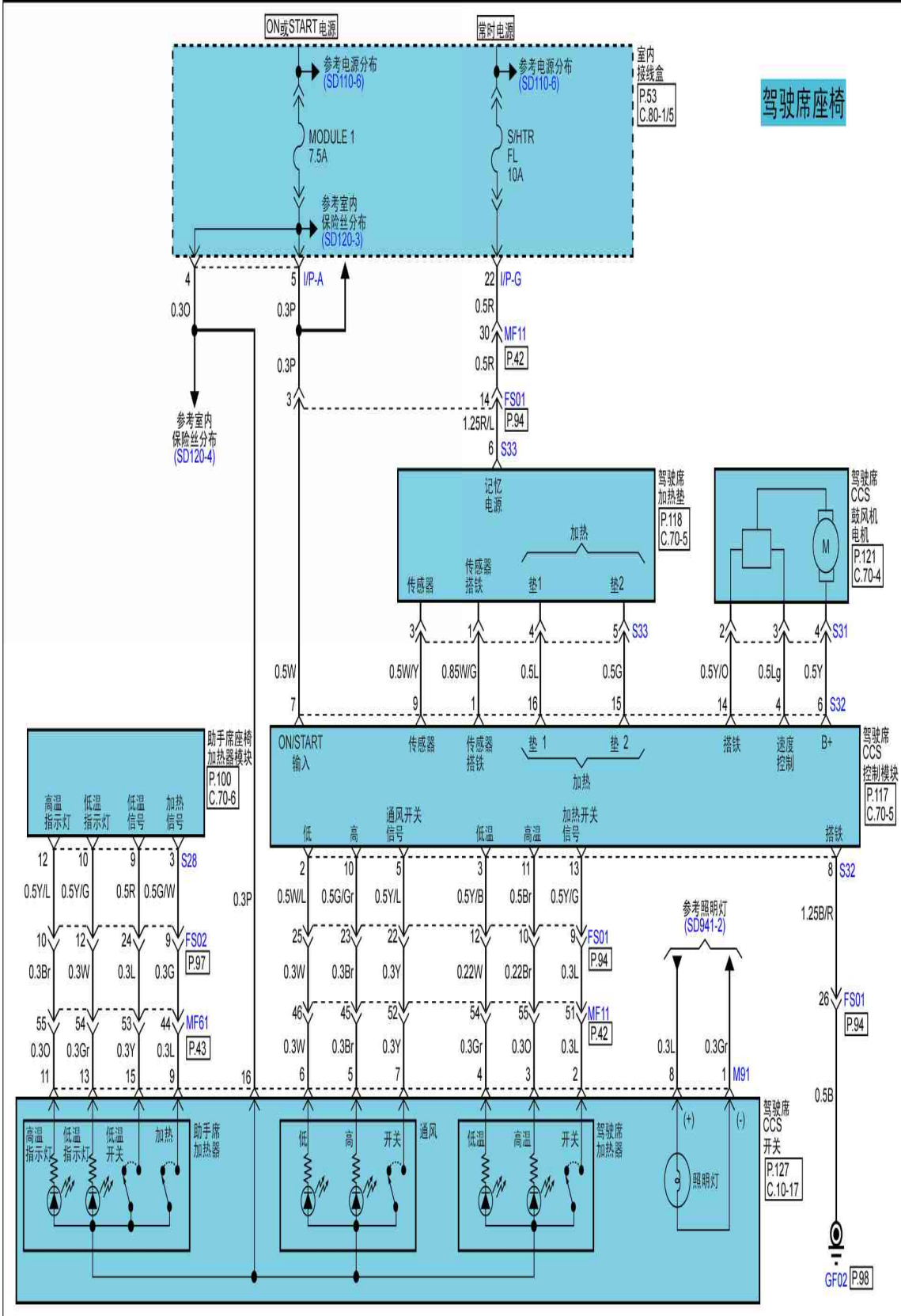
温度控制座椅控制系统 (1)
